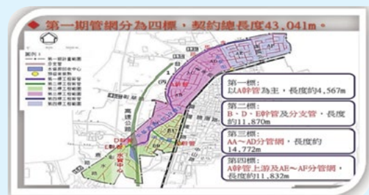
圖1-6 第一期污水管網分標示意圖
