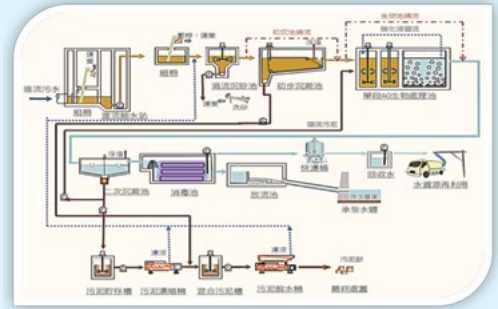
圖1-2處理流程圖
