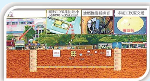
圖1-7管線推進示意圖
